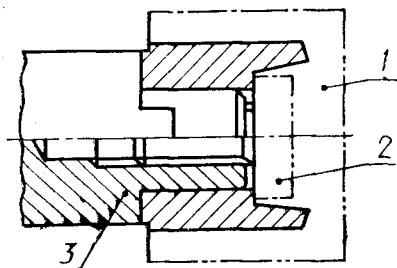
1—фреза; 2—стопорный винт; 3—центрирующая часть оправки
