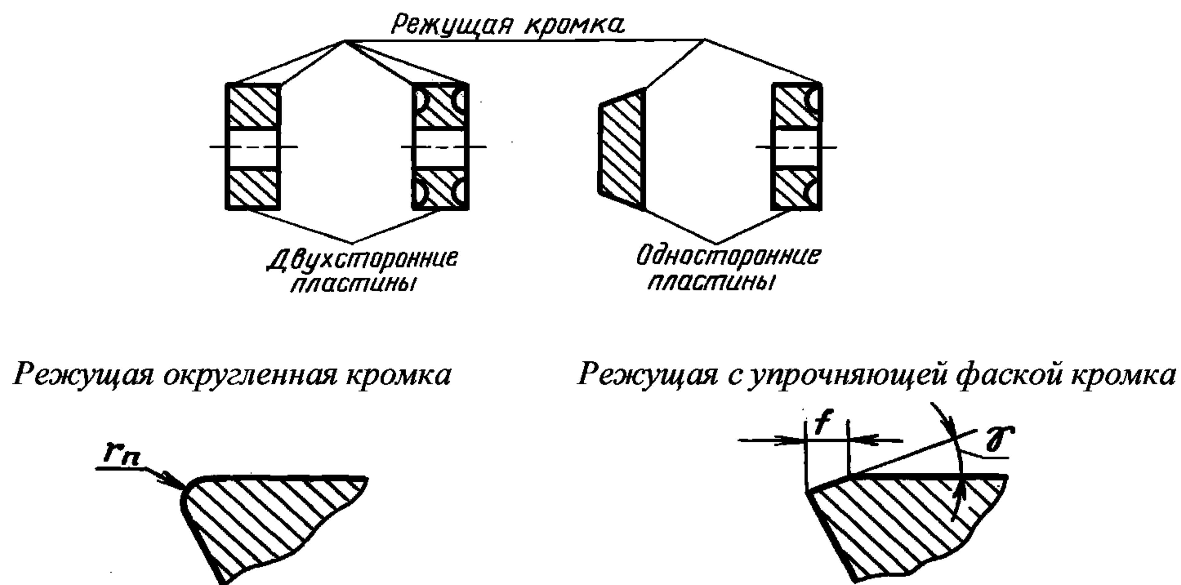
r_n — радиус округления режущей кромки; f — ширина упрочняющей фаски режущей кромки
